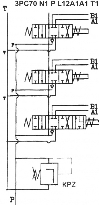
parallel circuit paralel dolaşım
