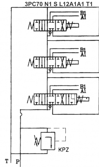
series circuit seri dolaşım
