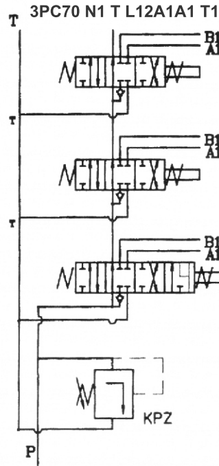
tandem circuit tandem dolaşım
