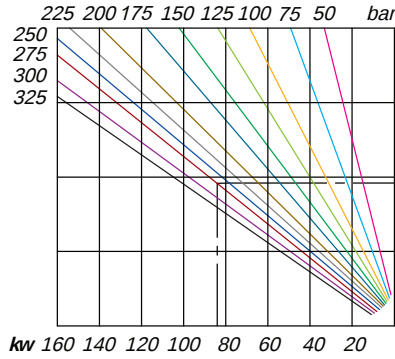
Emilmiş Güç - Absorbed Power
