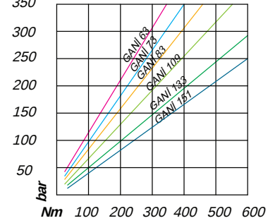
Giriş Torku - Input Torque
