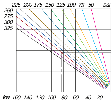
Emilmiş Güç - Absorbed Power
