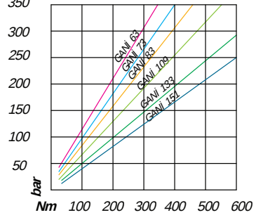
Giriş Torku - Input Torque
